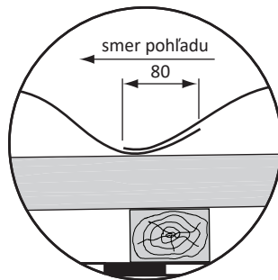
Detail 2.: Bočné prekrytie ľavého panelu pravým, nie naopak
